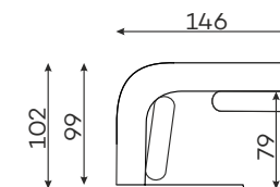
ELEMENT NAROŻNY ASYMETRYCZNY
